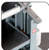
Mesa de cepillado de acero fundido sobre 4 cilindros roscados
