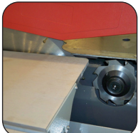
Hoja Ø 250 mm e incisor Ø 80 mm
