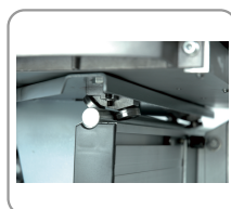
Slede voor plugboren met glijdsysteem op kogellagers
