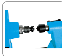
Aanpassing van de punten cm2 en meenemerstift met schroefdraad m33 x 3,5 mm
