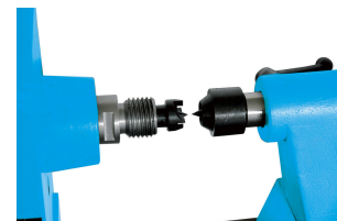
Kop in gietstaal, meenemerstift m33 x 3,5 mm
