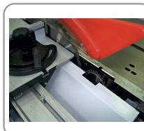
Zaagblad \varnothing 315 of \varnothing 250 mm, voorritsblad van \varnothing 100 mm
