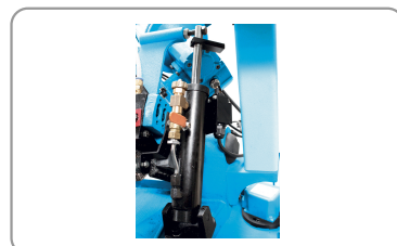
Afdaling van de boeg door hydraulische cilinder met regelbaar debiet
