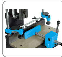
2 snel aanspanbare verticale persbalken en 1 glijdende horizontale persbalk
