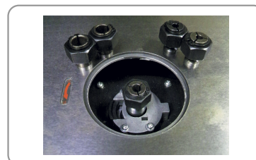
5 spantangen (6 - 6.35 - 8 - 12 - 12,7 mm)
