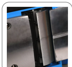
Arbre équipé de 2 mini-fers carbure réversibles.
