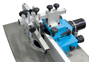
Freesbankgeleider met horizontale en verticale persbalken
