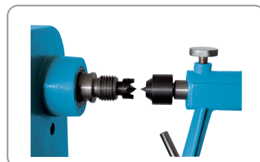
Meenemerstift met schroefdraad m33 x 3,5 mm
