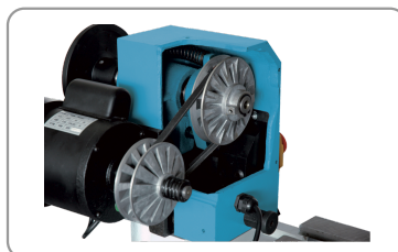
Motor met riem
