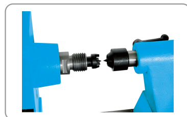
Aanpassing van de punten cm2 en meenemerstift met schroefdraad m33 x 3,5 mm
