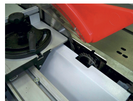
Zaagblad Ø 315 of Ø 250 mm, voorritsblad van Ø 100 mm
