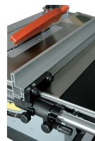
Geleider voor doorzagen in de lengte met micrometer afstelling
