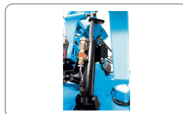
Afdaling van de boeg door hydraulische cilinder met regelbaar debiet
