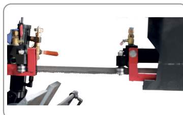
Aanpasbare en zeer nauwkeurige geleiding van het zaagblad met 8 punten rollen
