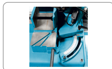
Drillboog draaibaar van 0° tot 60° links voor samengestelde sneden
