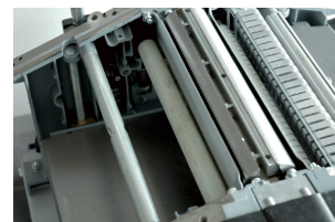
Aandrijvingsrollen voor de aanvoer van het stuk hout
