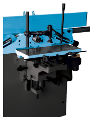
Optie pengatboormachine
