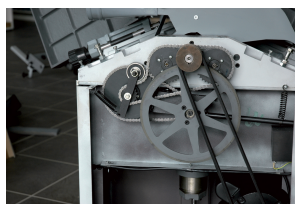
Kettingaandrijving, motoraandrijving met dubbele riem
