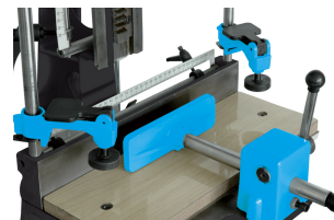
2 snel aanspanbare verticale persbalken en 1 glijdende horizontale persbalk
