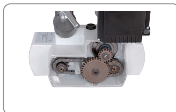
Kettingaandrijving
