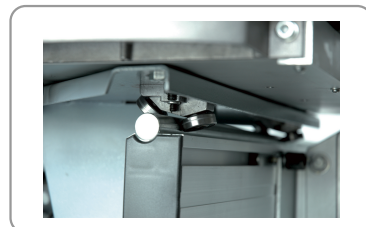
Slede voor plugboren met glijdsysteem op kogellagers
