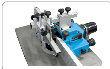
Freesbankgeleider met horizontale en verticale persbalken
