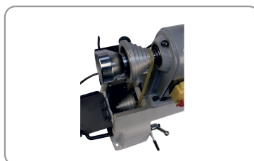
6 mechanische snelheden
