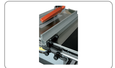
Geleider voor doorzagen in de lengte met micrometer afstelling
