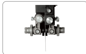
Geleider voor het bovenste en onderste blad met rollen
