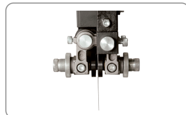
Geleider voor het bovenste en onderste blad met rollen
