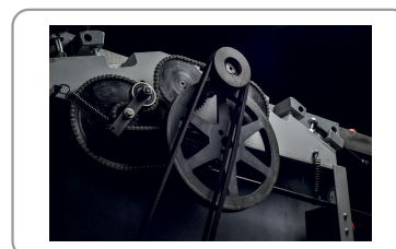
Kettingaandrijving, motoraandrijving met dubbele riem
