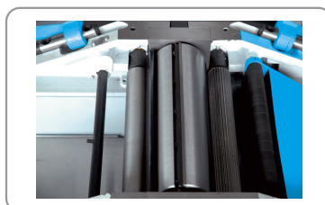
Aandrijvingsrollen voor de aanvoer van het stuk hout
