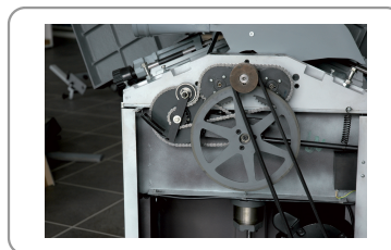
Kettingaandrijving, motoraandrijving met dubbele riem
