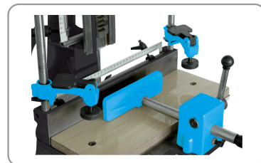
2 snel aanspanbare verticale persbalken en 1 glijdende horizontale persbalk
