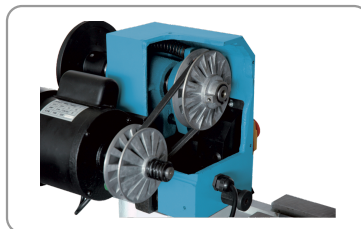
Moteur avec courroie et poulies coniques
