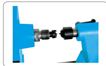
Alignement des pointes cm2 et broche dentrainement fileté m33 x 3,5 mm
