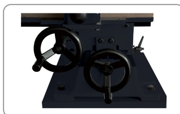
Double chariotage latéral et longitudinal sur queue daronde
