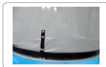
Sangle à feillard + attache de maintien du sac
