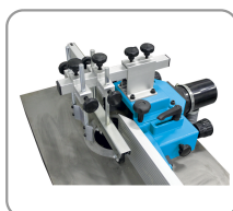
Guide de toupie avec presseurs horizontal et vertical.
