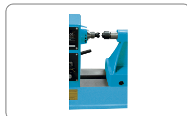
Broche entraînement cm2 filetée m33 x 3,5 mm
