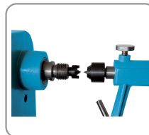
Broche dentrainement cm2 fileté m33 x 3,5 mm
