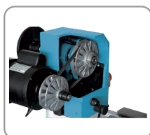
Moteur avec courroie et poulies coniques
