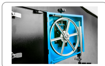
Volants en fonte d'aluminium équilibrés et contacteurs de sécurité
