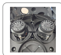
2 moteurs à refroidissement by-pass montés en parallèle
