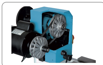
Moteur avec courroie et poulies coniques
