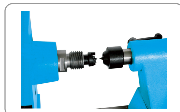
Alignement des pointes cm2 et broche d'entraînement filetée m33 x 3,5 mm
