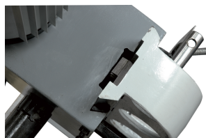
Coulissement de la tête sur queue d'aronde
