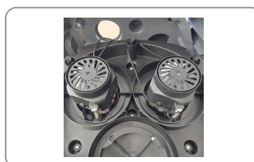
2 moteurs à refroidissement by- pass montés en parallèle
