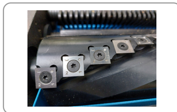
Arbre hélicoïdal à plaquettes carbure standards
