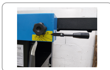
Réglage de la table d'entrée par levier excentrique
