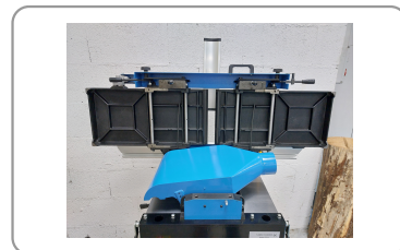
Ouverture des tables en une seule opération
