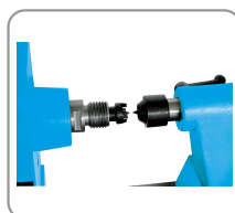
Allineamento punte cm2 e mandrino di trasmissione filettato m33 x 3,5 mm
