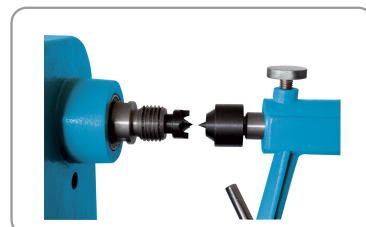
Mandrino di trasmissione cm2 filettato m33 x 3,5 mm
