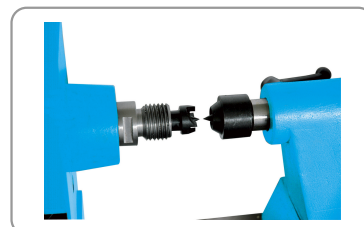
Allineamento punte cm2 e mandrino di trasmissione filettato m33 x 3,5 mm
