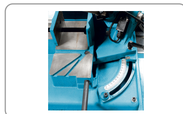
Archetto orientabile da 0° a 60° a sinistra per tagli in squadra
