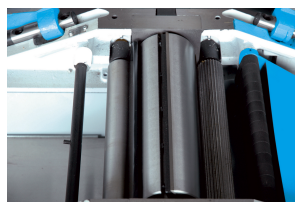
Rulli guida Ø 40 mm per l'avanzamento dell'elemento in legno, albero da 95 mm a 4 ferri
