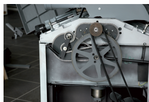
Alimentazione rulli a catena, trasmissione motore a doppia cinghia
