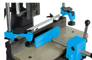
2 pressori verticali a serraggio rapido e 1 pressore orizzontale scorrevole
