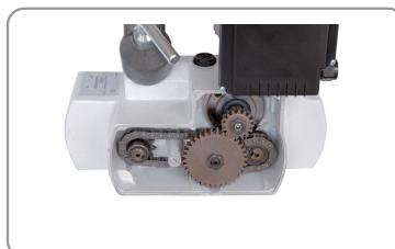
Trasmissione a catena
